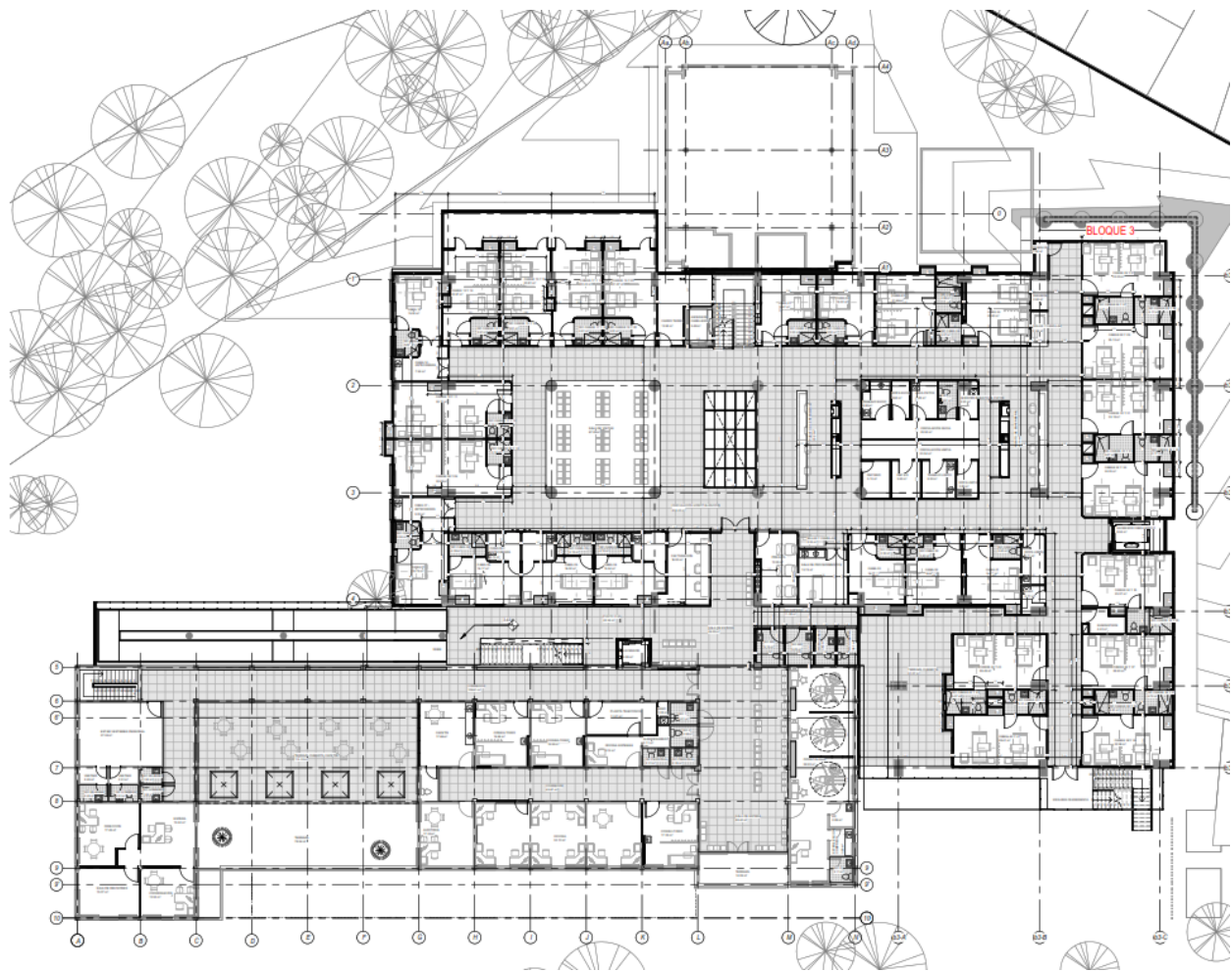
Planta nivel 3
