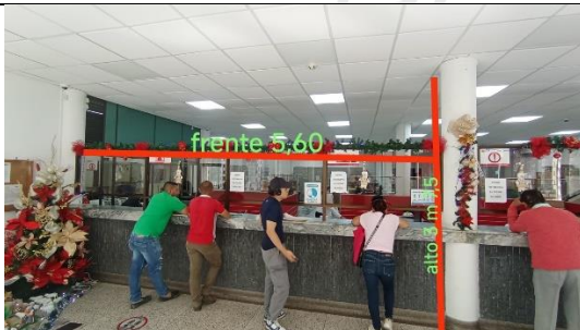
DIVISION EN VIDRIO LAMINADO 3+3 M2 - MESON TIPO MOSTRADOR DE ATENCION AL PUBLICO DE ALTURA ENTRE 0.90 A 1.10 - DIVISIONES MODULARES PISO TECHO, ALTO 2,20 m M2
