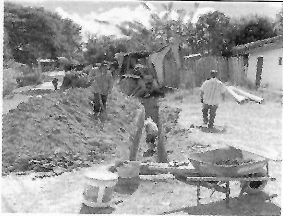
Lecho de arena y/o grava
