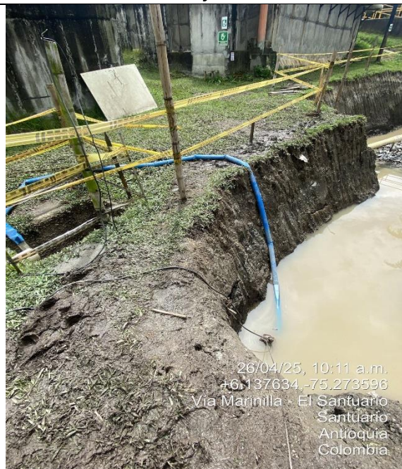
Fotografía 3. Manejo de aguas de infiltración, subterráneas y nivel freático mediante bombas sumergibles.
