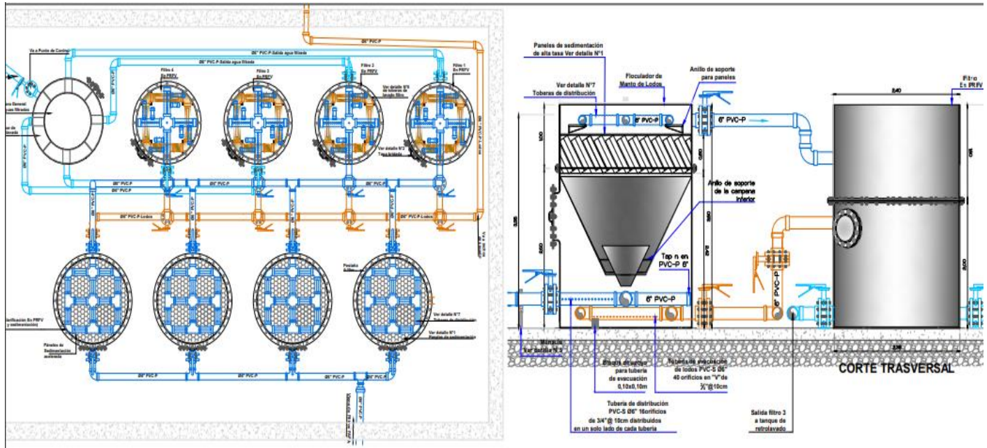
Ilustración 4: Detalle planta-perfil sedimentadores+floculadores y tanques de filtración rápida.
