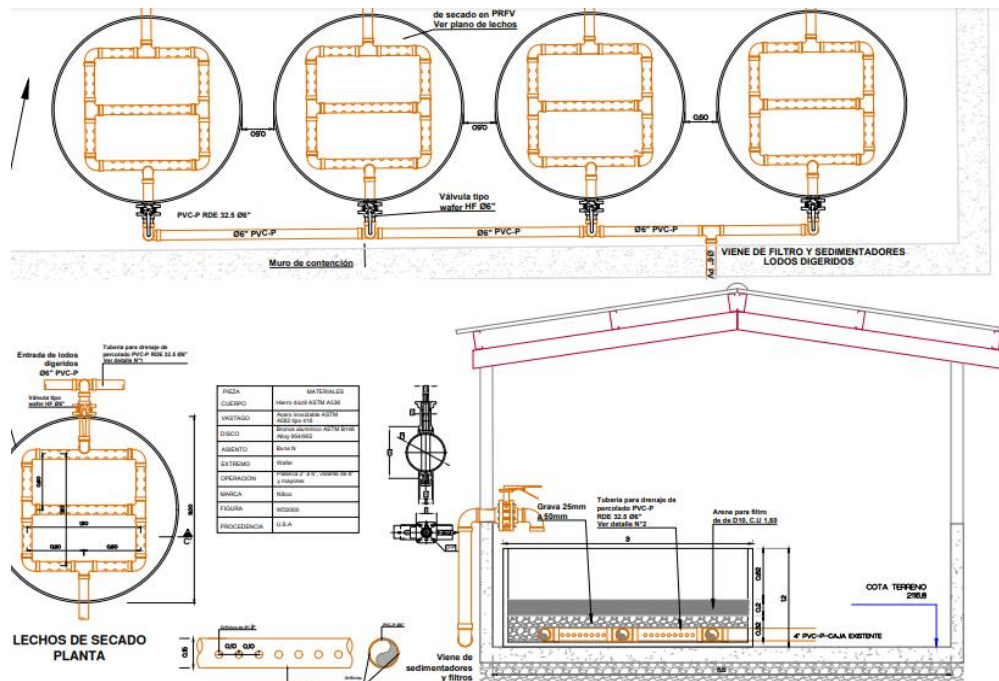
Ilustración 5: Detalle planta-perfil de lechos de secado.
