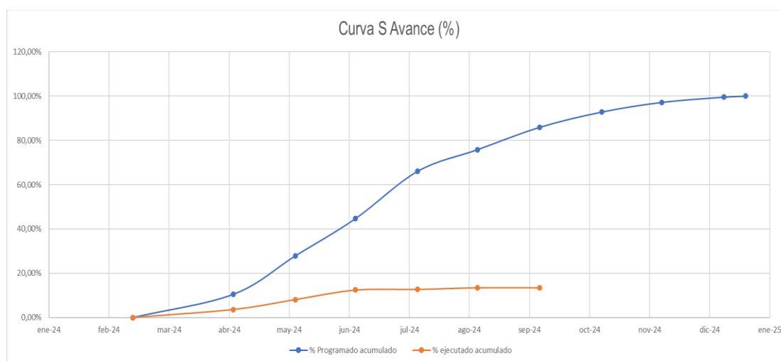
Ilustración 48. Curva S – Avance Físico Porcentual del presente período
