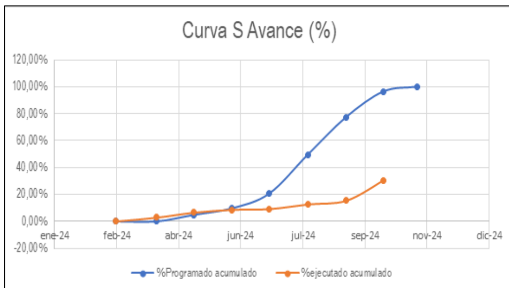
Ilustración 5. Curva S – Avance Físico Porcentual del presente período
