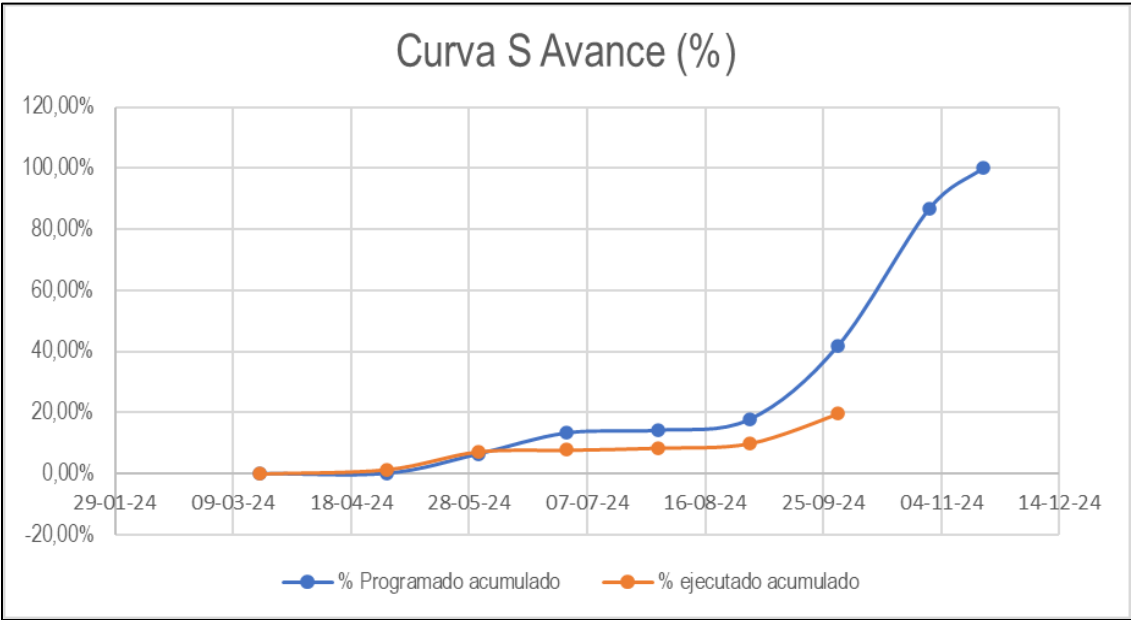
Ilustración 7. Curva S – Avance Físico Porcentual del presente período Fuente: Elaboración propia.
