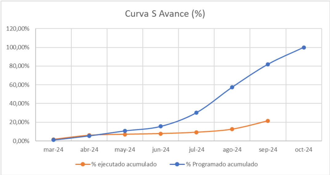
Ilustración 40. Curva S – Avance Físico porcentual del presente período Fuente: Elaboración propia.
