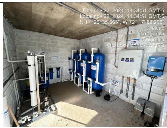
Fotografía 2. Planta de osmosis inversas.
