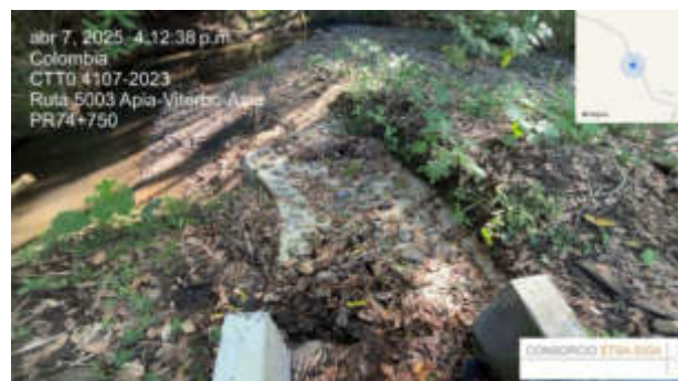
Figura 9 Entrega de agua con enrocado PR74+750
