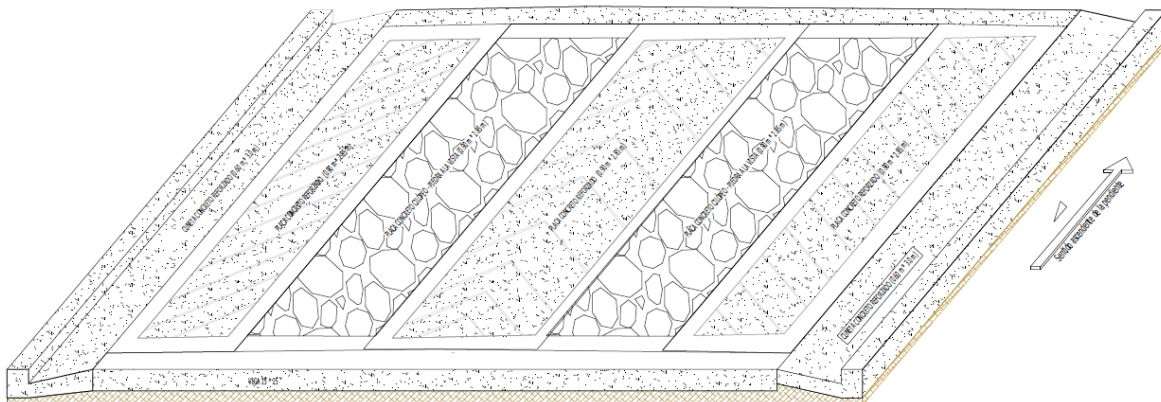
Ilustración 1, Isometría modelo placa Huella sobre ancho y sección de cuneta tipo "L"
