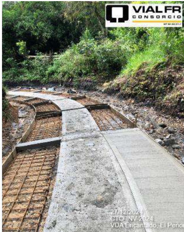
CONCRETO CICLOPEO Y PARRILLAS DE HUELLA
