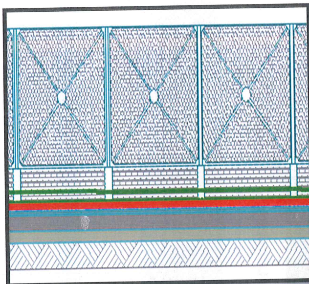
Detalle concreto ciclópeo, viga de cimentación y pedestales
