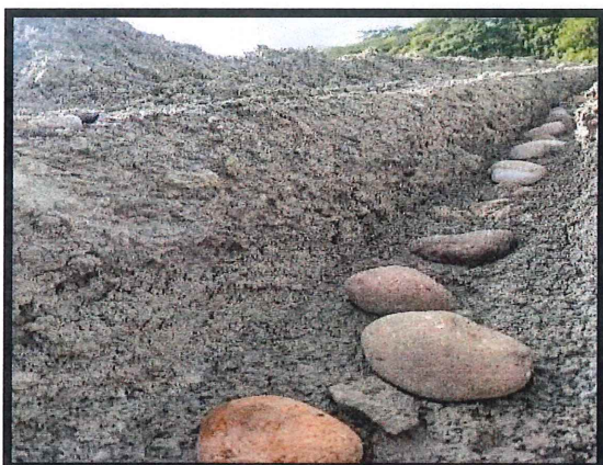
5.1 Concreto ciclópeo 2500 psi
