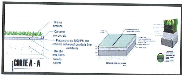
Detalle de cuenta perimetral - Cárcamo
