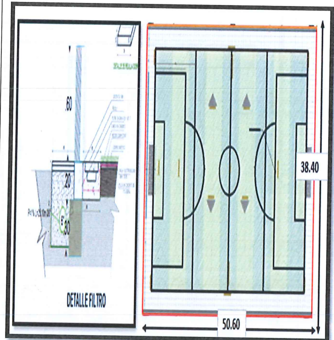
Detalle filtros laterales externos
