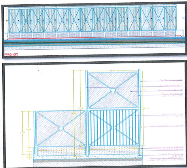
Detalle placa de piso en concreto de 3000 PSI
