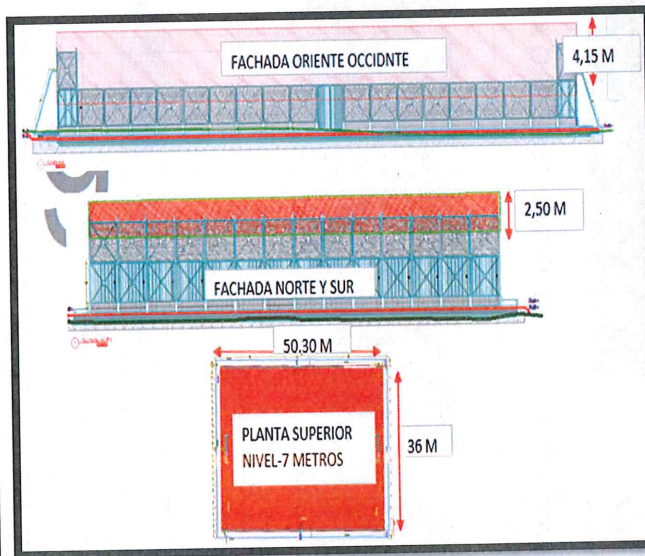
Detalle cerramiento metálico Módulos cerramiento 2,5x2,5 m en malla eslabonada
