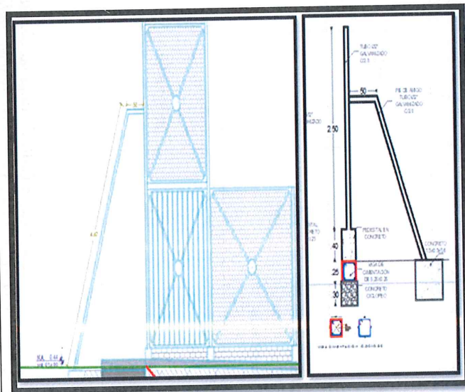
Detalle de cerramiento metálico Módulos cerramiento 2,5x2,5 m en ángulo 1 1/2"x1/8 con varilla de 5/8"
