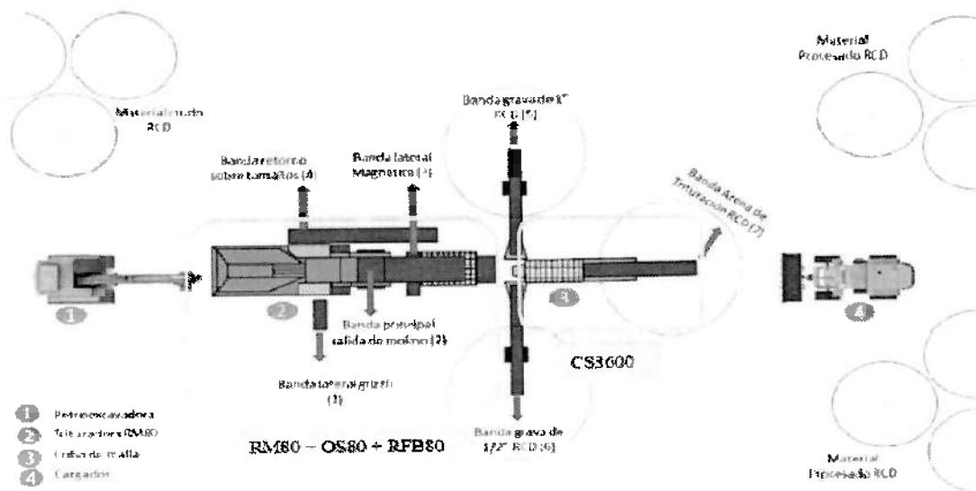
Ilustración No. 5. Diagrama del proceso de trituración – Línea productiva Cemex Colombia S.A. – Planta de Tratamiento y Aprovechamiento de RCD
