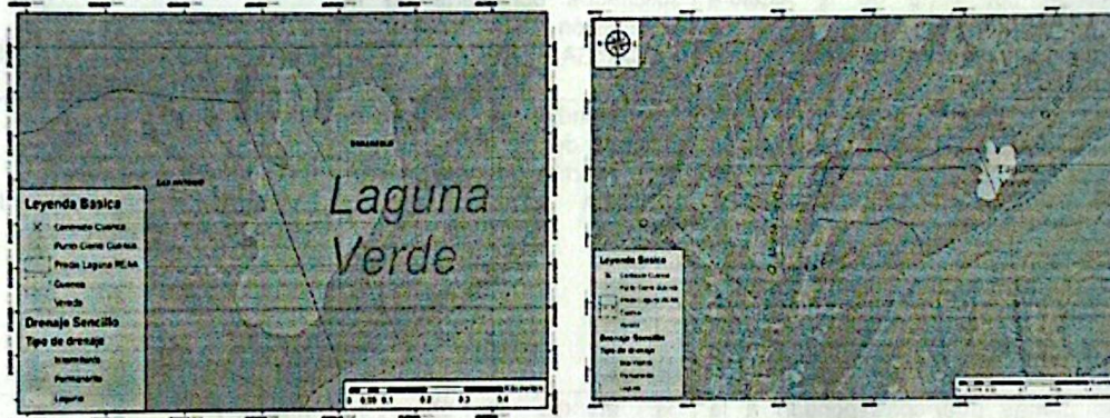
Figura 3 Cuerpos hídricos identificados en el área de estudio
