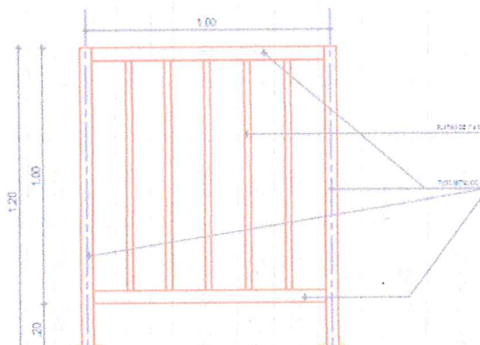
Ilustración No. 32 –Suministro e instalacion de baranda metálica en tubo de 2", incluye soldadura, thinner, anticorrosivo, pintura y todas las actividades necesarias para la correcta ejecución de la actividad.
