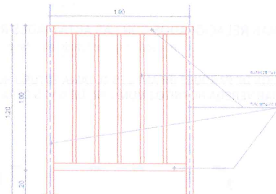
Ilustración No. 3 –Suministro e instalación de baranda metálica en tubo de 2", incluye soldadura, thinner, anticorrosivo, pintura y todas las actividades necesarias para la correcta ejecución de la actividad.
