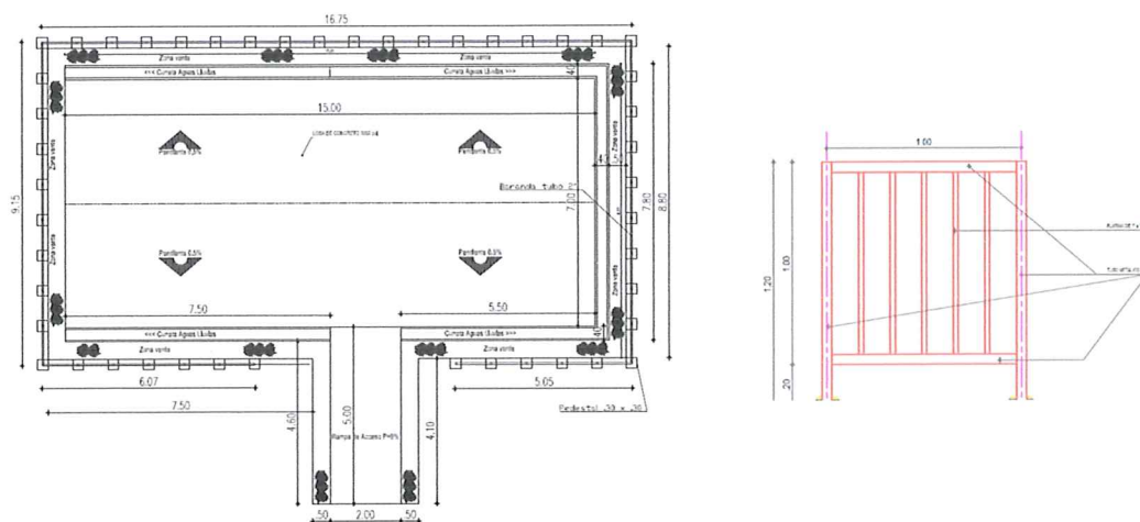
Ilustración No. 3 – Vista en planta y en perfil de la actividad de instalación de baranda metálica en tubo de 2".
