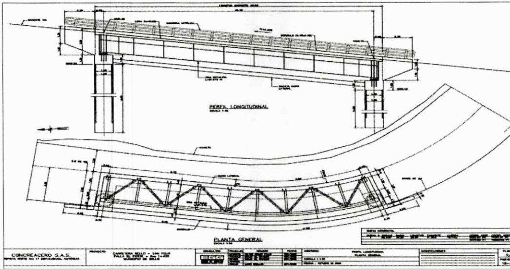
Detalle de diseño y Planta general punto crítico El Poste
