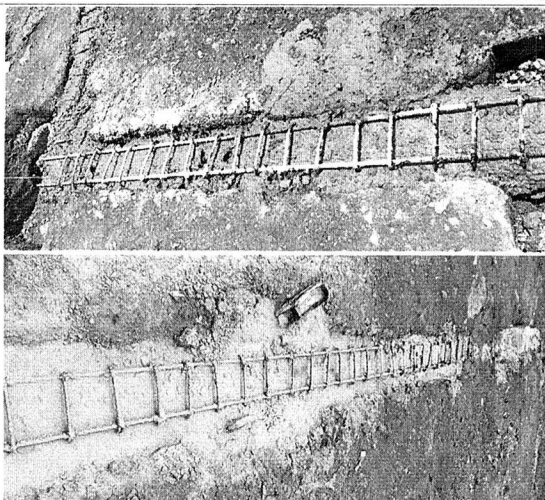
Malos procesos constructivos
