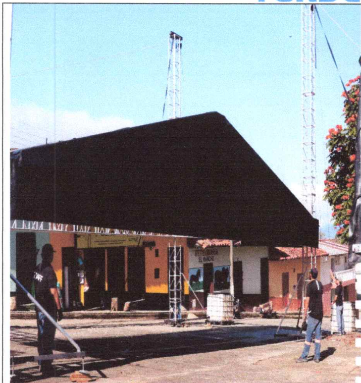
TECHO TIPO PABELLON
