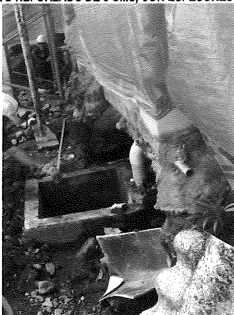
Cajas de inspección de aguas residuales - 29 al 31 de octubre del 2024.
