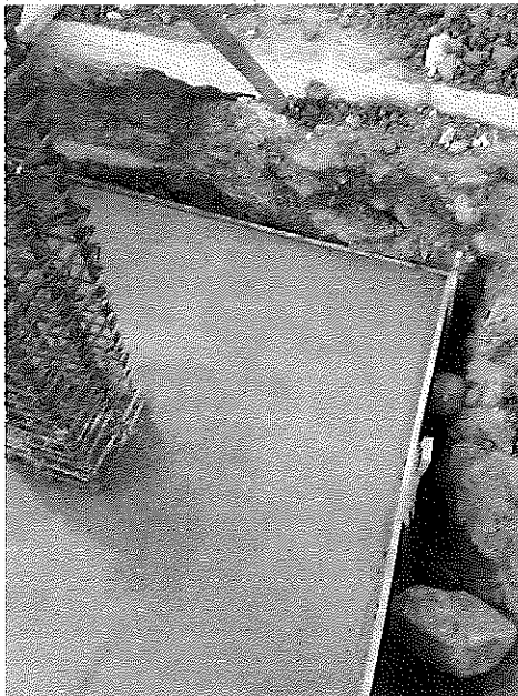
Construcción zapatas en concreto 3000 PSI – 07 al 15 de octubre del 2024.
