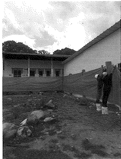
Construcción cerramiento perimetral - 29 de octubre del 2024.
