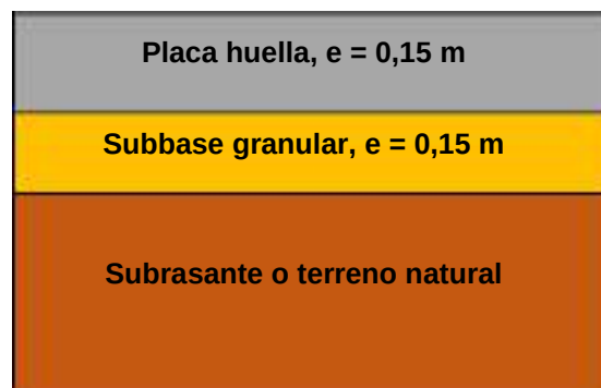
Ilustración. Espesores de la placa huella.
