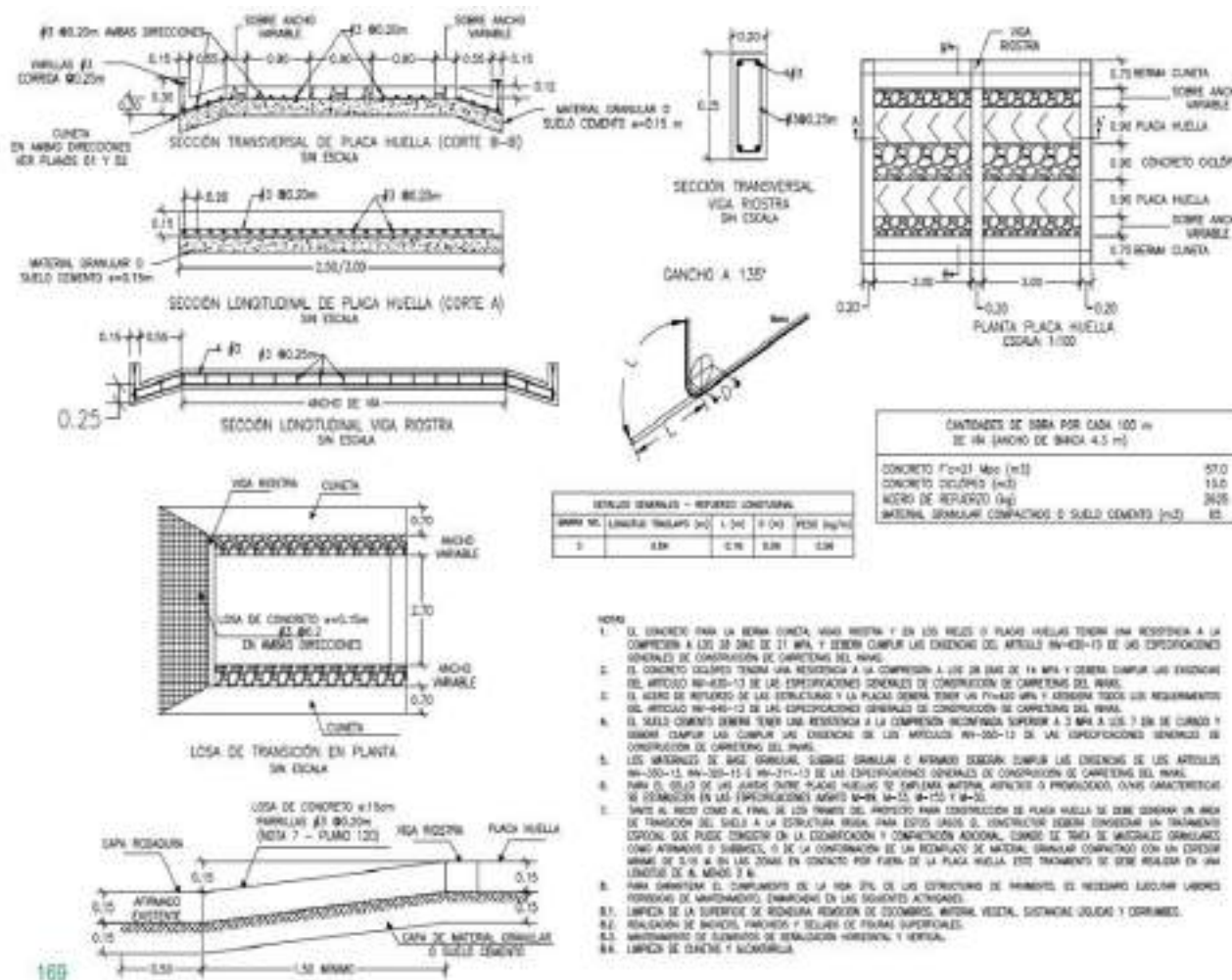
Ilustración. Detalles técnicos de diseño de la placa huella (Cartilla de INVÍAS).
