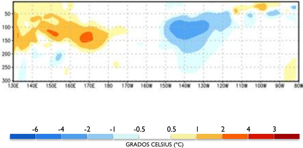
Anomalías de la Temperatura Subsuperficial del Mar (°C), pentada centrada en el 27 de julio 2025. Fuente: NOAA
