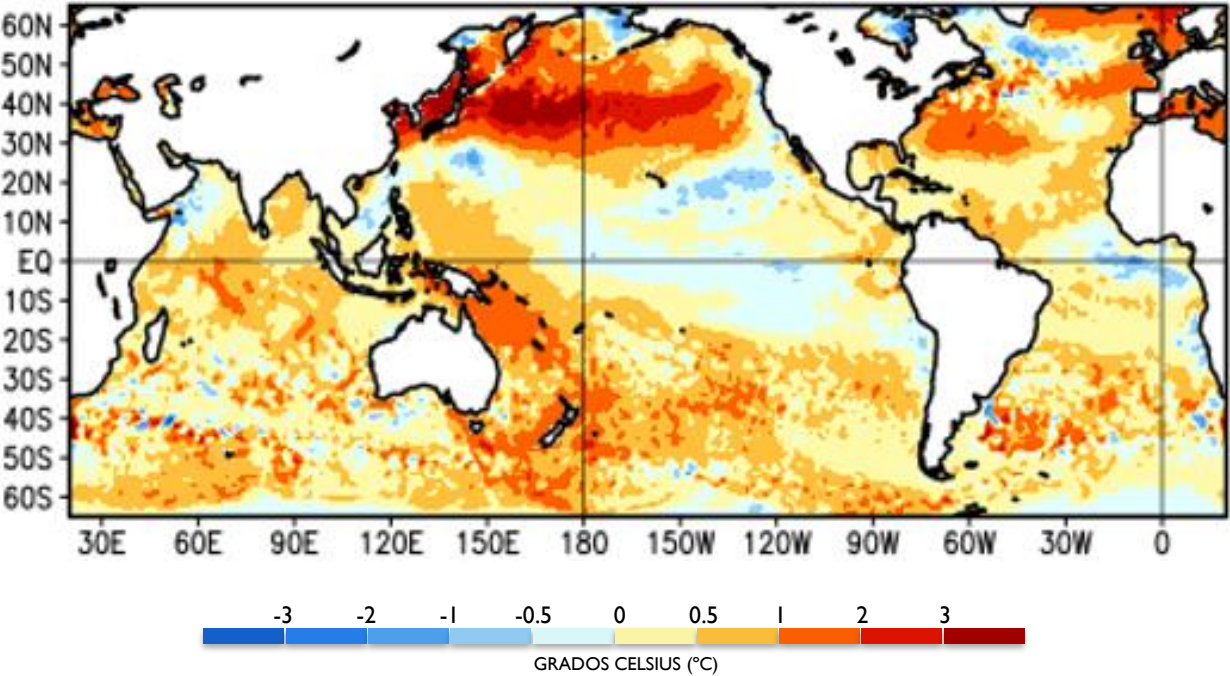
Promedio de las Anomalías de la Temperatura Superficial del Mar (°C) entre el 06 de julio y el 02 de agosto de 2025. Fuente: NOAA
