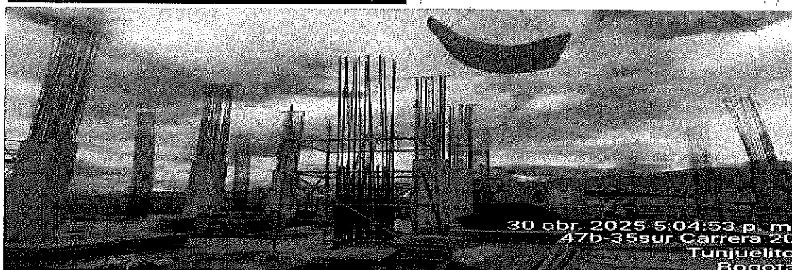
Zona B y Voladizo eje F-G. En armado y fundido de columnas piso 4 a piso 5
