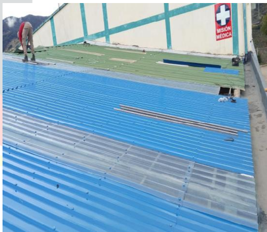
Instalación de teja en polycarbonato
