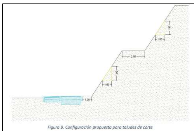
Configuración Propuesta para Taludes.
