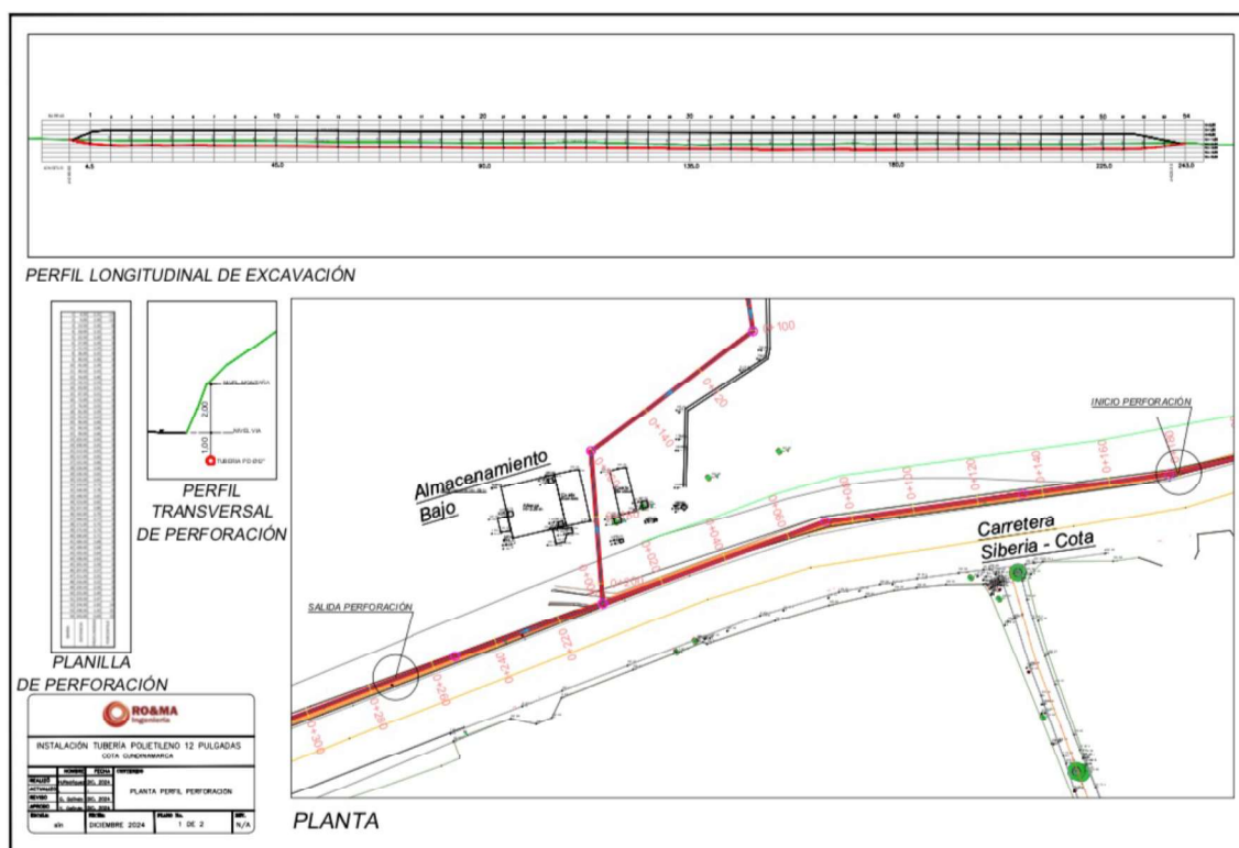
Diseño Perforación Horizontal Dirigida (PHD)
