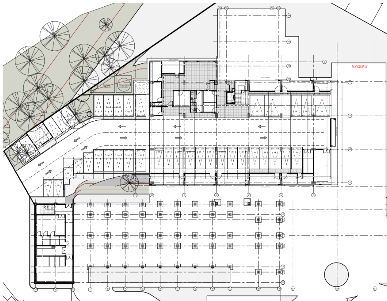
Planta Cubiertas
