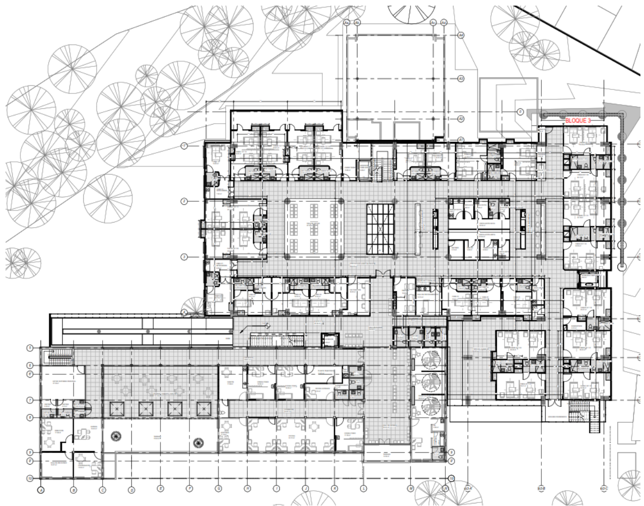
Planta nivel 3
