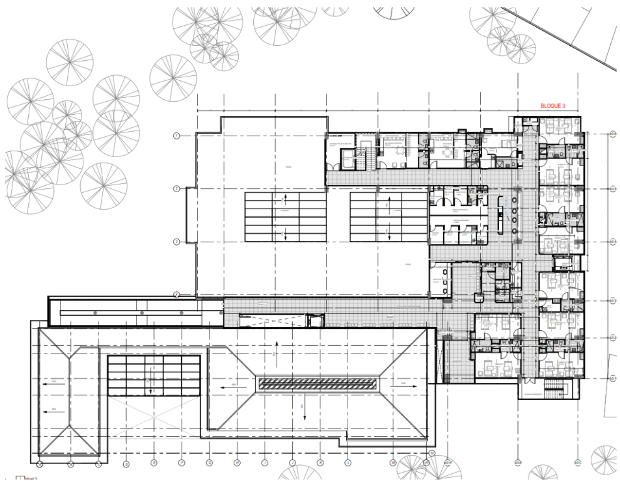
Planta nivel -1
