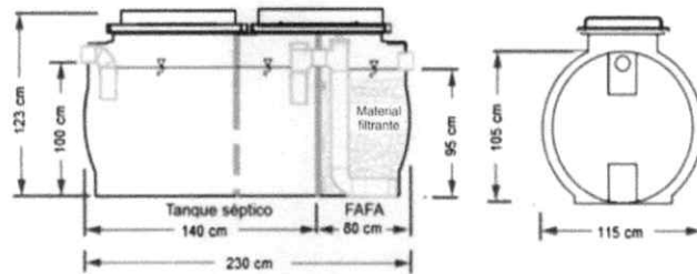
GRAFICO No. 1. SISTEMA SÉPTICO INTEGRADO.
