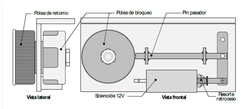
Figura 4. imagen demostrativa mecanismo de bloqueo
