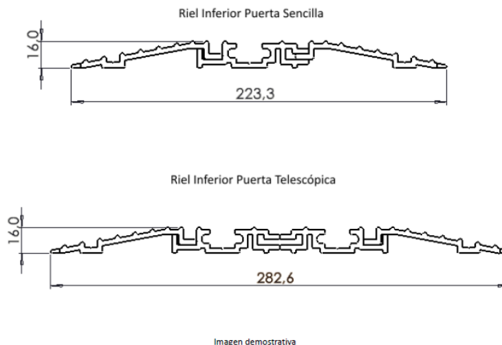
Figura 2. Corte lateral sistema de guías y rampas. Parte superior esquema para puerta de dos (2) hojas, parte inferior esquema para puerta (4) hojas, imagen demostrativa.
