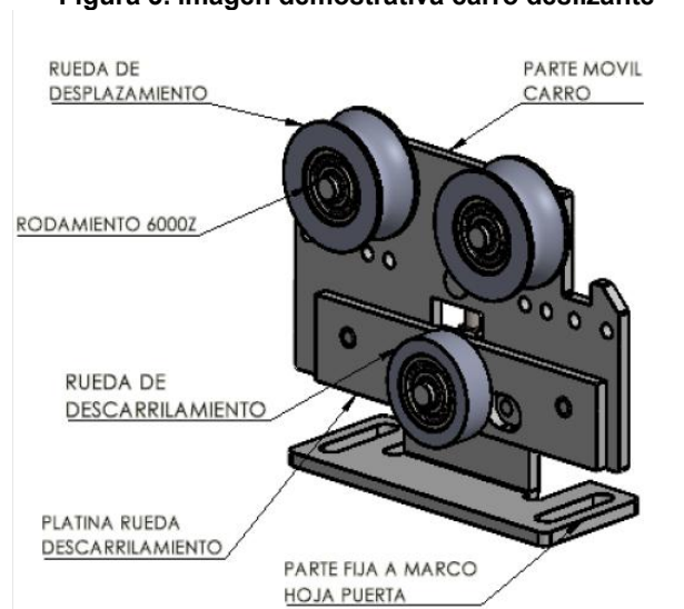
Figura 3. imagen demostrativa carro deslizante
