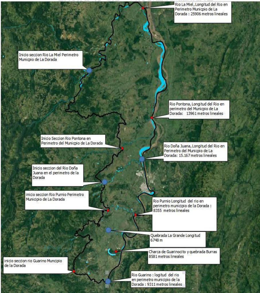
Longitud dentro del perímetro del municipio , Río Guarinó tributario al Río Magdalena
