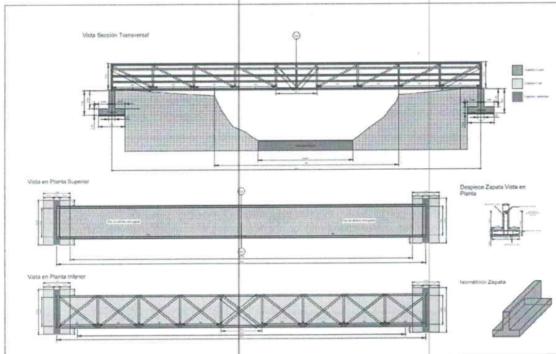
Ilustración 2 Esquema Mejoramiento y Reforzamiento Estructural Para el Puente Peatonal.
