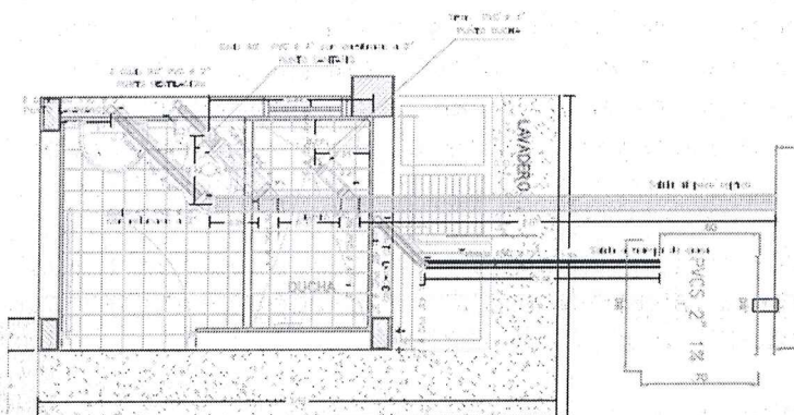
DETALLE INSTALACIONES SANITARIAS
