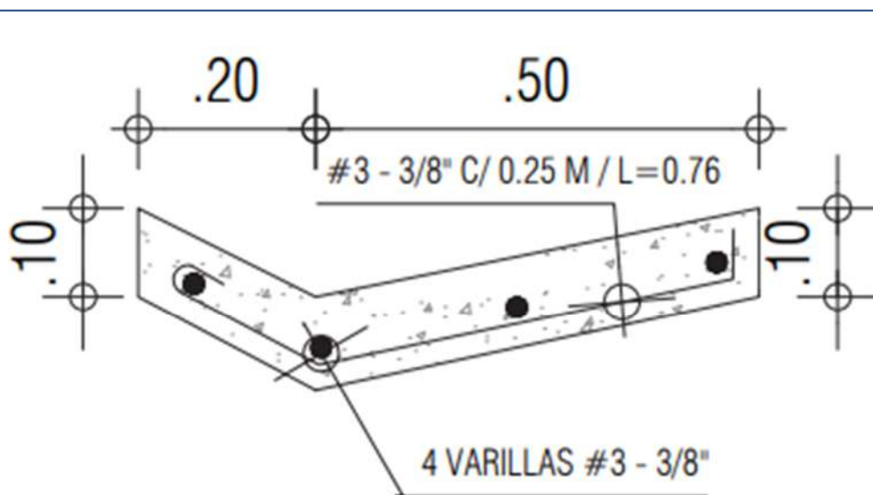
DETALLE CUNETA TIPO 2
