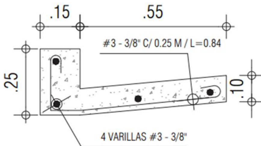
DETALLE CUNETA TIPO 1
