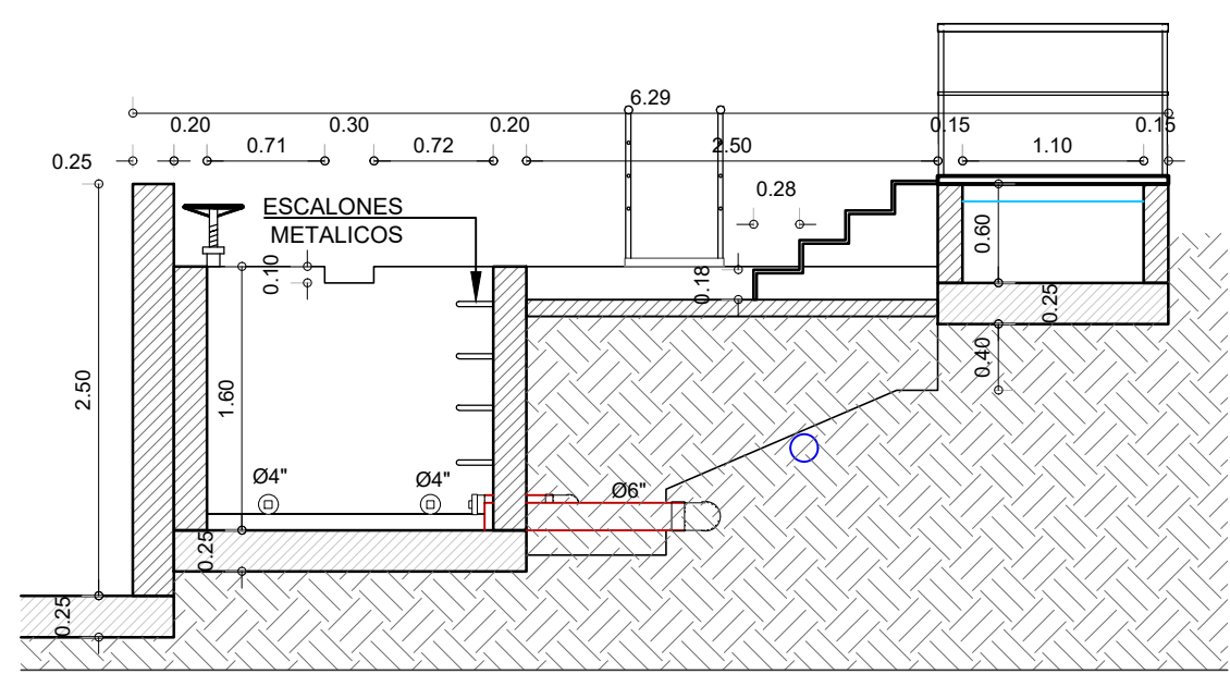
CORTE D-D ESCALA 1:50
