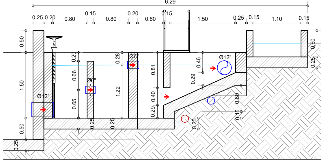
VORTE C-C ESCALA 1:50
