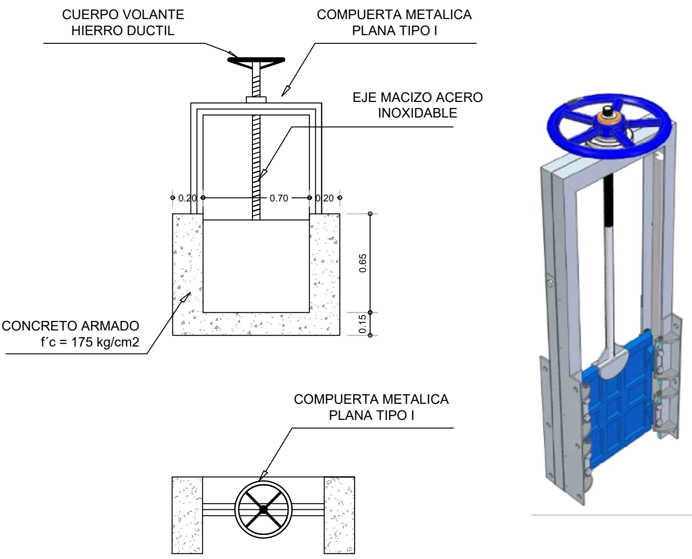
DETALLE COMPUERTA METÁLICA SIN ESCALA
