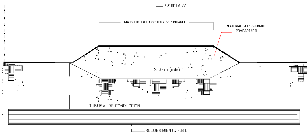
Figura 12 Esquema de cruce por zanjado a cielo abierto en vías
