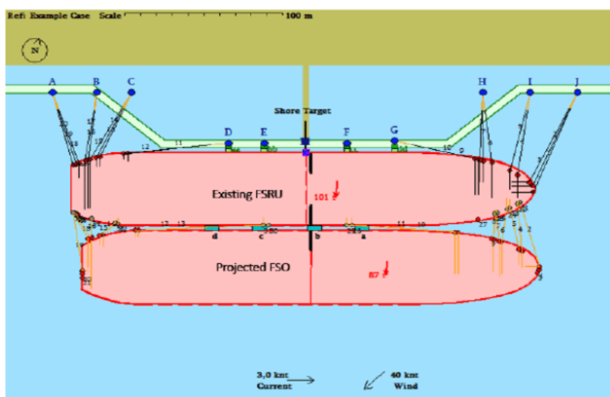
Figura 5 Esquema amarre flotante entre buques
