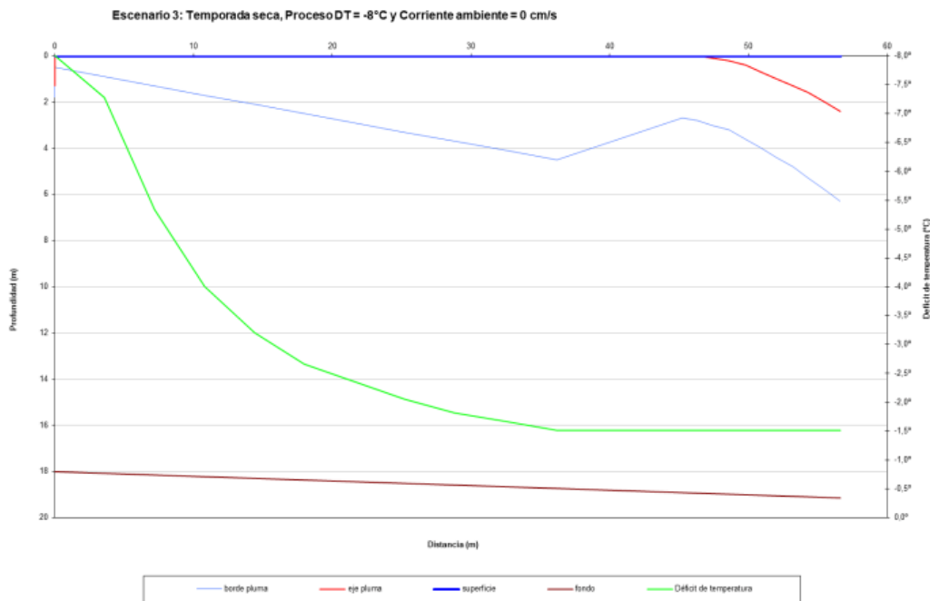
Figura 16. Resultados del modelo de dispersión de temperatura para el escenario 3 Fuente: Modelación de un vertimiento térmico en la bahía de Cartagena., SPEC LNG., 2021
