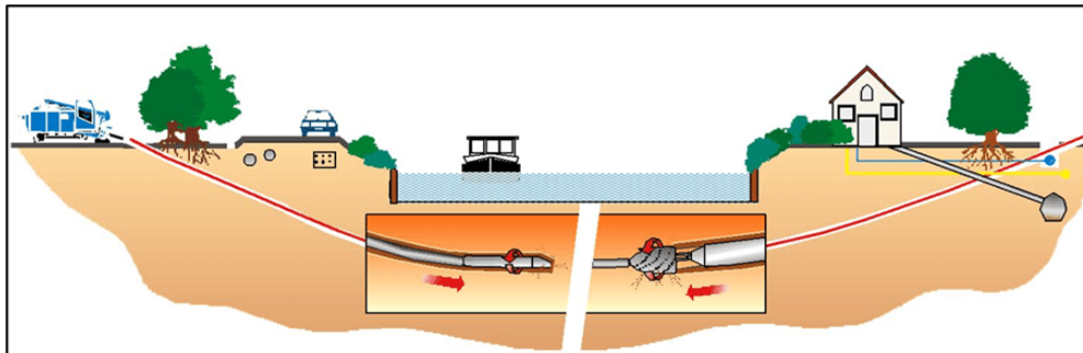
Figura 8 5 Esquema de Procedimiento Constructivo Perforación Horizontal Dirigida
