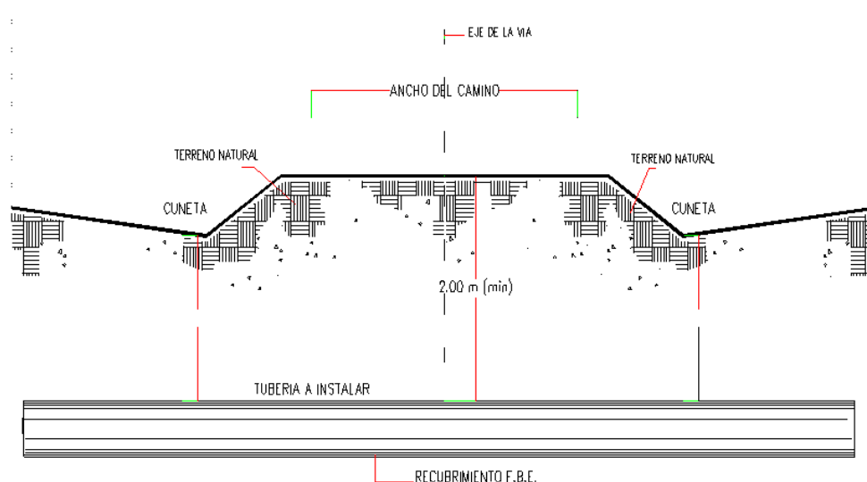
Figura 13 Esquema de cruce por zanjado a cielo abierto en vías Fuente: SPEC, 2024
