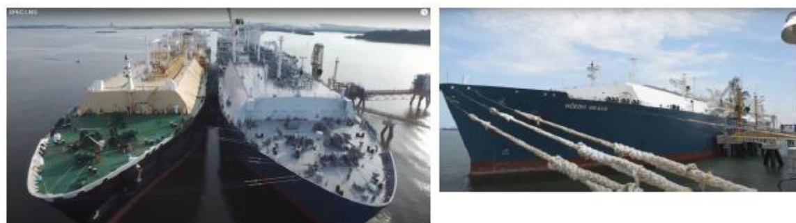
Figura 6 Amarre flotante entre buques
