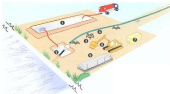
Figura 6 Esquema Plataforma de Salida Perforación Horizontal
