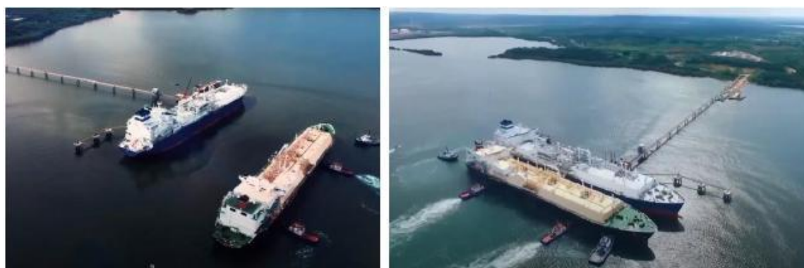
Figura 4 Aproximación de buque guiado con remolcadores a FSRU existente Fuente: SPEC, 2025
