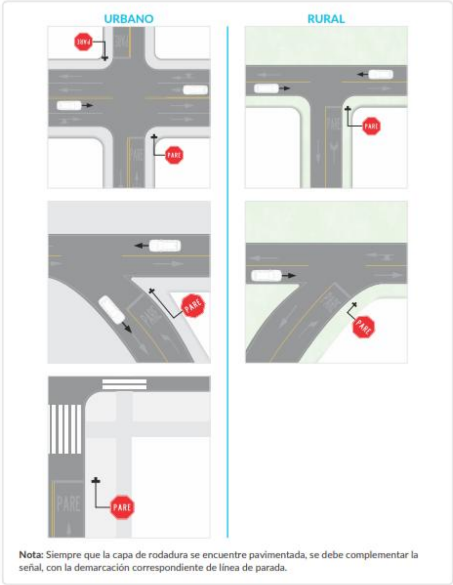
Figura 2-17. Ubicación típica de señal SR-01 PARE
