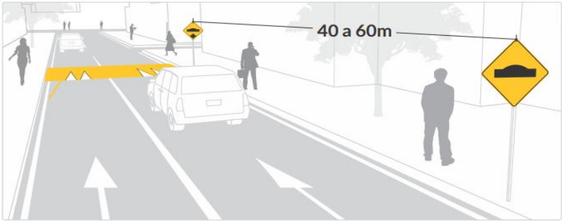
Figura 2-32. Señalización para resalto
