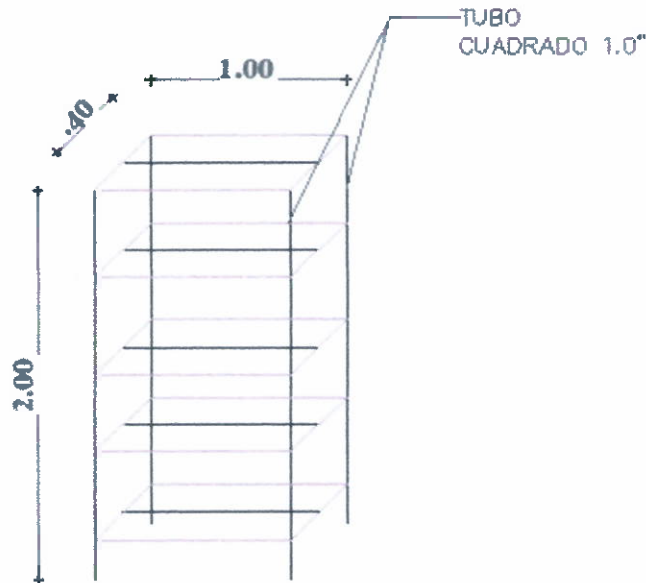
Ilustración 3. Esquema de las dimensiones de los estantes
