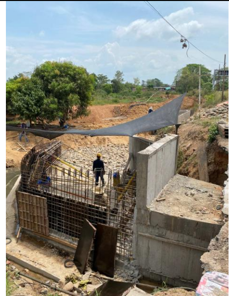
FOTO 34. 2025-03-05 CONTINUACIÓN DE ENCOFRADO DE PARTE BAJA DE LA ALETA IZQUIERDA AGUAS DEBAJO DE BOX CULVERT K0+500 VÍA SAN PABLO – SIMITÍ
