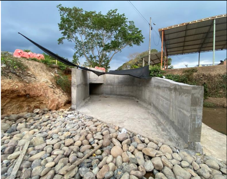
FOTO 145. 2025-03-16 ESTADO GENERAL DE LAS OBRAS DEL BOX CULVERT K0+500 VÍA SAN PABLO - SIMITÍ
