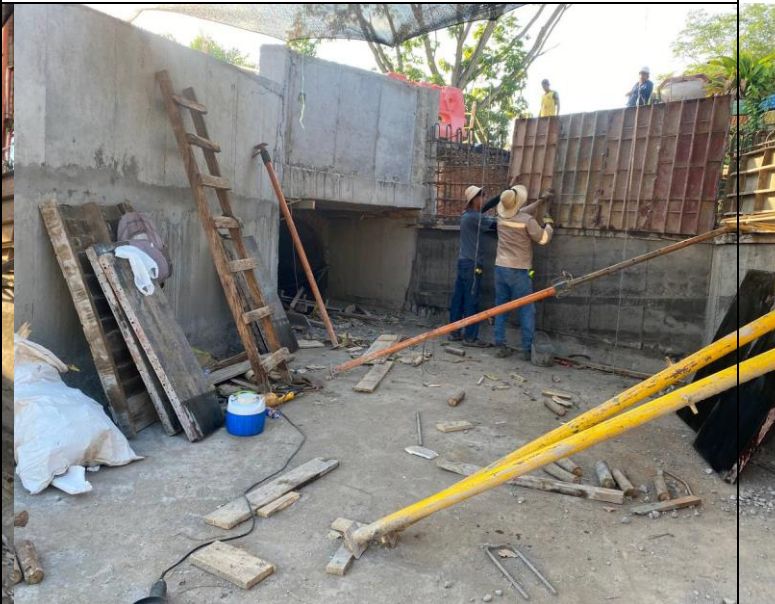
FOTO 84. 2025-03-07 DESENCOFRADO DE PARTE INFERIOR DE ALETA IZQUIERDA. SE LLEVA A CABO ENCOFRADO DE LA PARTE SUPERIOR DE LA ALETA IZQUIERDA AGUAS ABAJO DE BOX CULVERT K0+500 VÍA SAN PABLO – SIMITÍ
