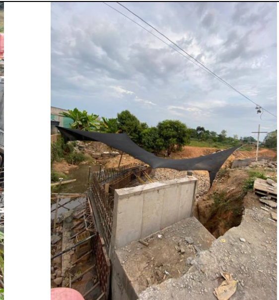
FOTO 60. 2025-03-06 FUNDIDA DE PARTE INFERIOR DE ALETA IZQUIERDA AGUAS ABAJO DE BOX CULVERT K0+500 VÍA SAN PABLO – SIMITÍ, CON CONCRETO DE 4000 PSI CON ADITIVO IMPERMEABILIZANTE Y APLICACIÓN DE ANTISOL
