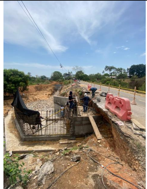
FOTO 4. 2025-03-01 DESENCOFRADO DE PARTE SUPERIOR DE LA ALETA DERECHA AGUAS DEBAJO DE BOX CULVERT K0+500 VÍA SAN PABLO – SIMITÍ. CONTINUACIÓN DE ENCONFRADO DE MURO PANTALLA EN LA PARTE SUPERIOR DE LA ESTRUCTURA DE TRANSICIÓN.
