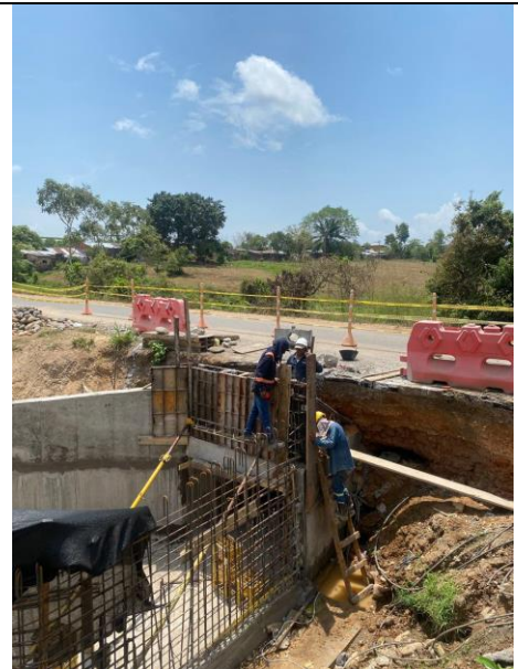
FOTO 2. 2025-03-01 DESENCOFRADO DE PARTE SUPERIOR DE LA ALETA DERECHA AGUAS DEBAJO DE BOX CULVERT K0+500 VÍA SAN PABLO – SIMITÍ. CONTINUACIÓN DE ENCONFRADO DE MURO PANTALLA EN LA PARTE SUPERIOR DE LA ESTRUCTURA DE TRANSICIÓN.
