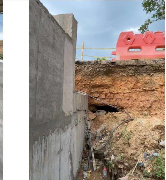
FOTO 148. 2025-03-16 ESTADO GENERAL DE LAS OBRAS DEL BOX CULVERT K0+500 VÍA SAN PABLO - SIMITÍ
