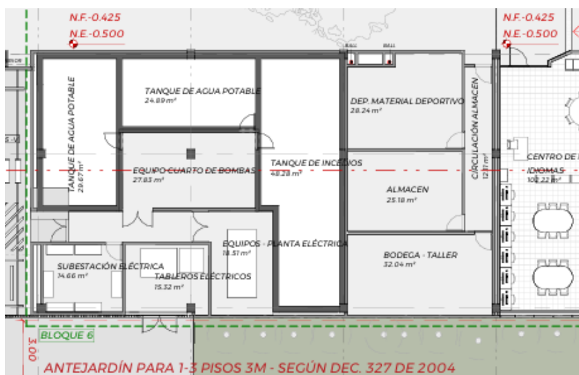
Imagen 3. Implantación original de los tanques en piso 1 bloque 6
