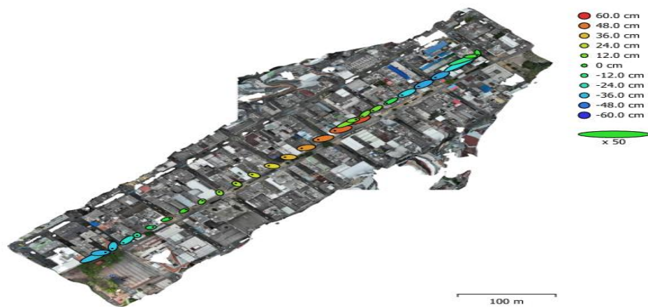
Fig. 3. Posiciones de cámaras y estimadores de error. El color indica el error en Z mientras el tamaño y forma de la elipse representan el error en XY. Posiciones estimadas de las cámaras se indican con los puntos negros.
