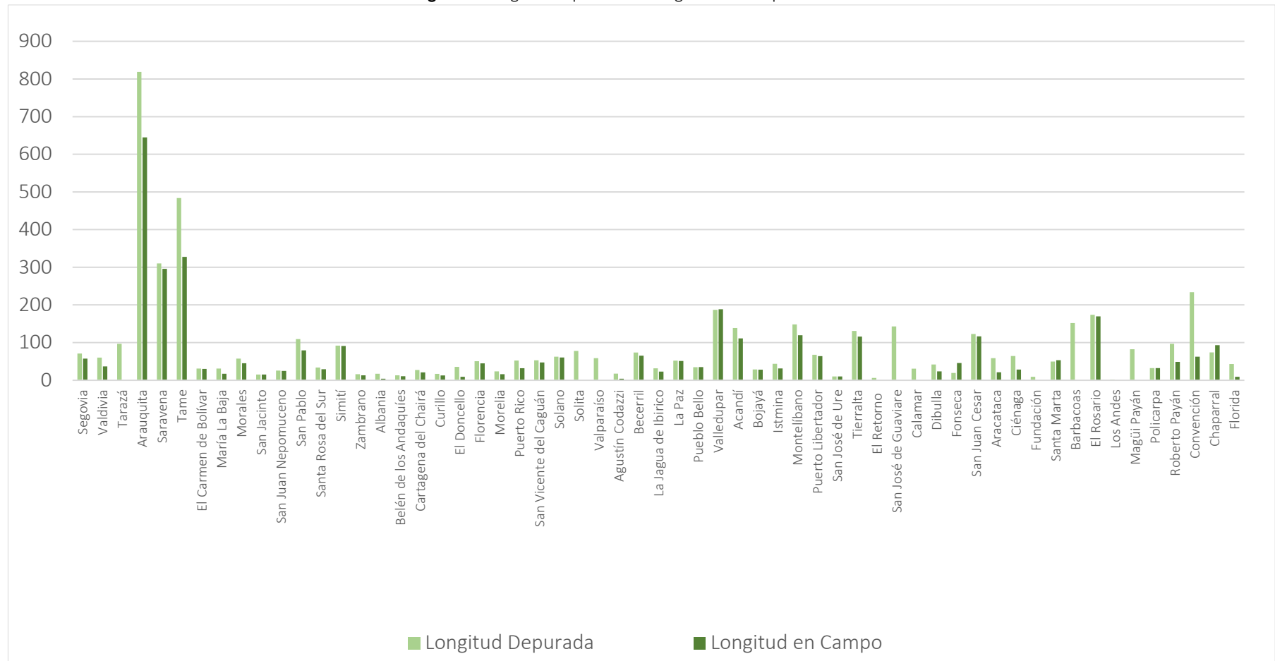
Figura 2. Longitud Depurada vs Longitud en Campo
