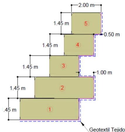
Ilustración 6. Figura representativa de muro en Geocontenedor. Fuente: Propia.
