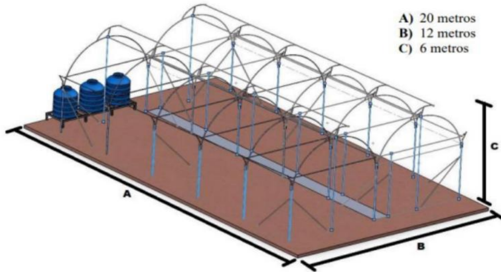
Medidas de la Estructura Invernadero en su Largo, Ancho y Altura
