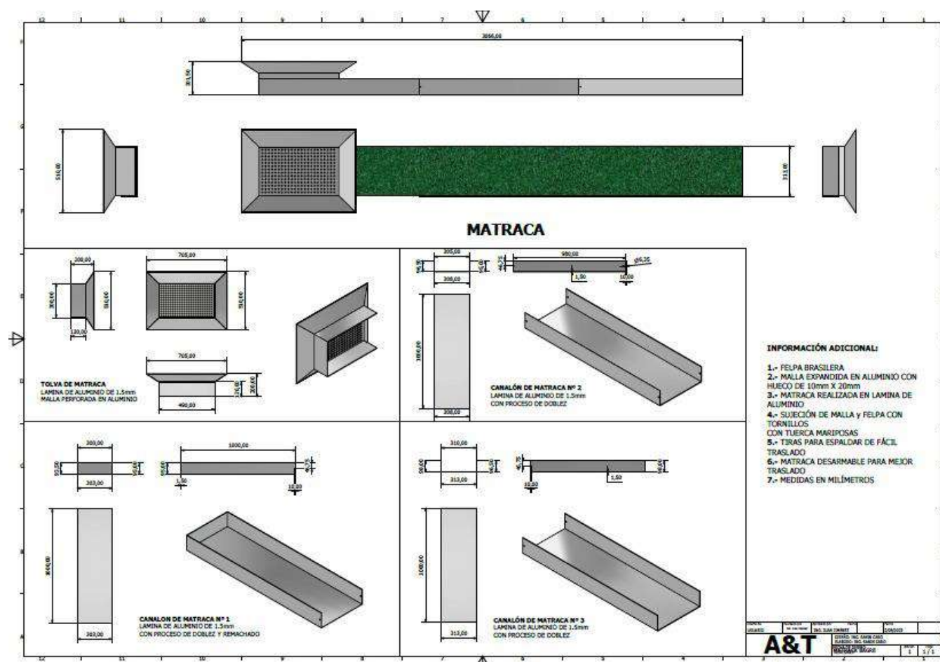
Ilustración 1. Especificaciones y diseño Matraca Sluice Plegable
