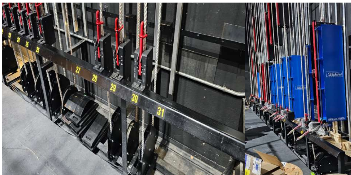
Imagen 3 y 4. Proceso de instalación y pruebas ítem 2 calle contrapesada
