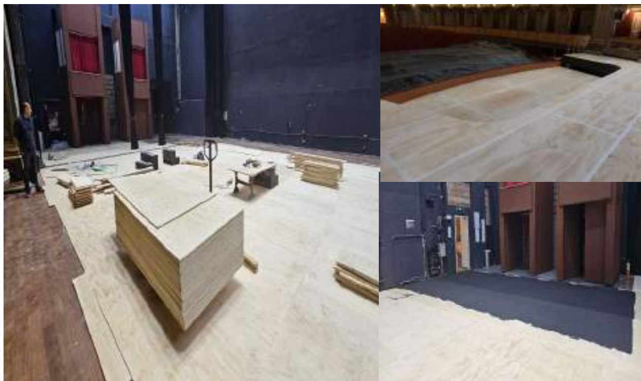
Imagen 3, 4 y 5. Proceso de instalación ítem 29
