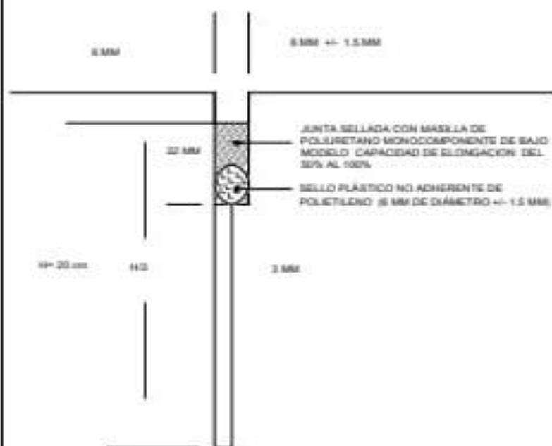
DETALLE CONSTRUCCIÓN JUNTA LONGITUDINAL
