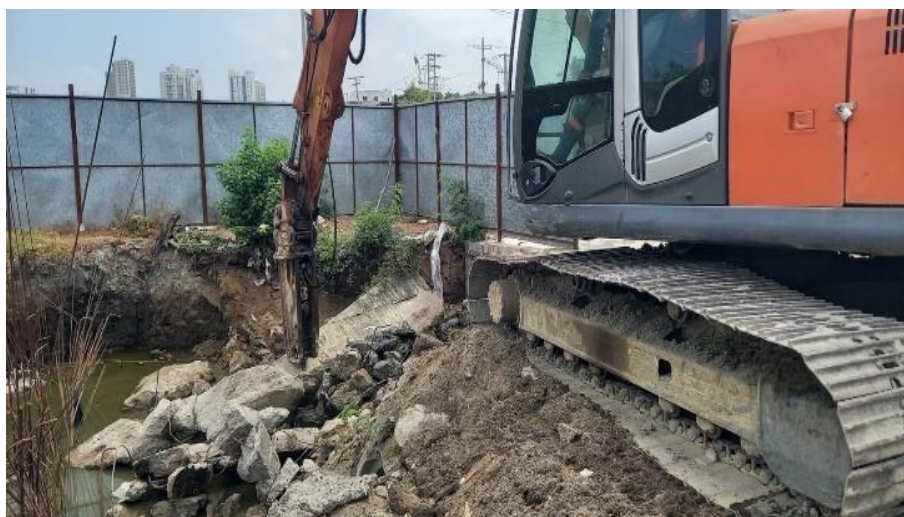
Ilustración 42. Demolición estructura de concreto box coulvert existente
