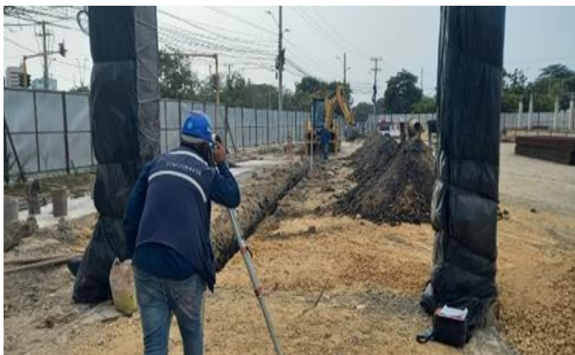
Ilustración 16. Localización y replanteo cerramiento externo
