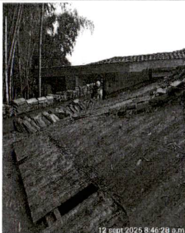
Retiro de teja de barro
