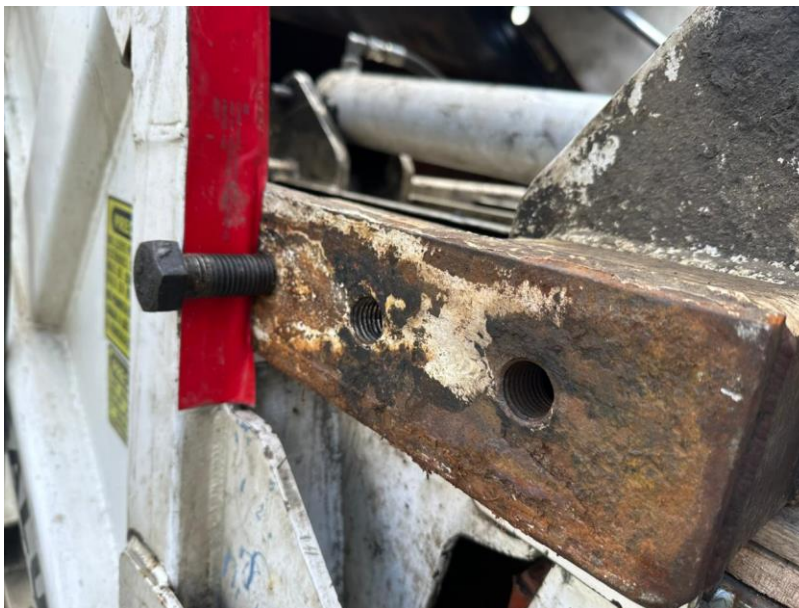
Desarme de guía para porta calzos y movimiento del sistema
