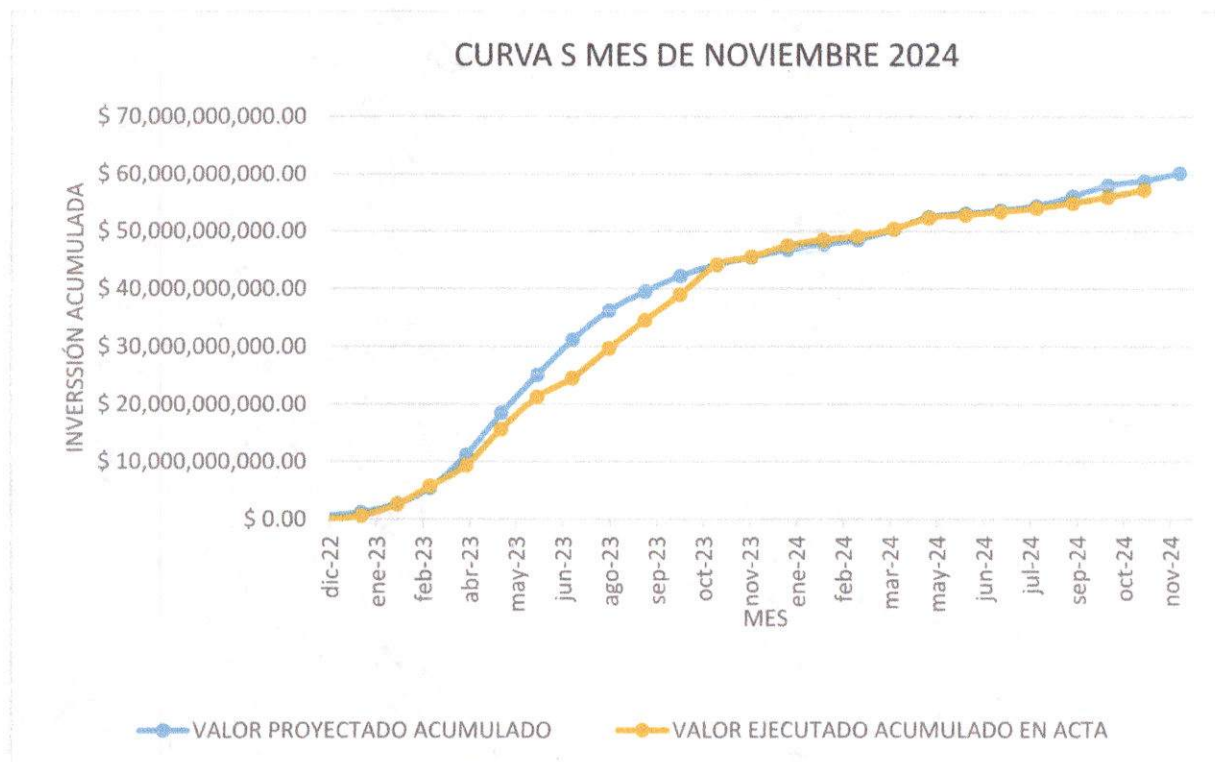
Figura 6. Curva S
