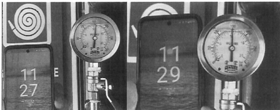
Ilustración 4 Monitoreo de presión
