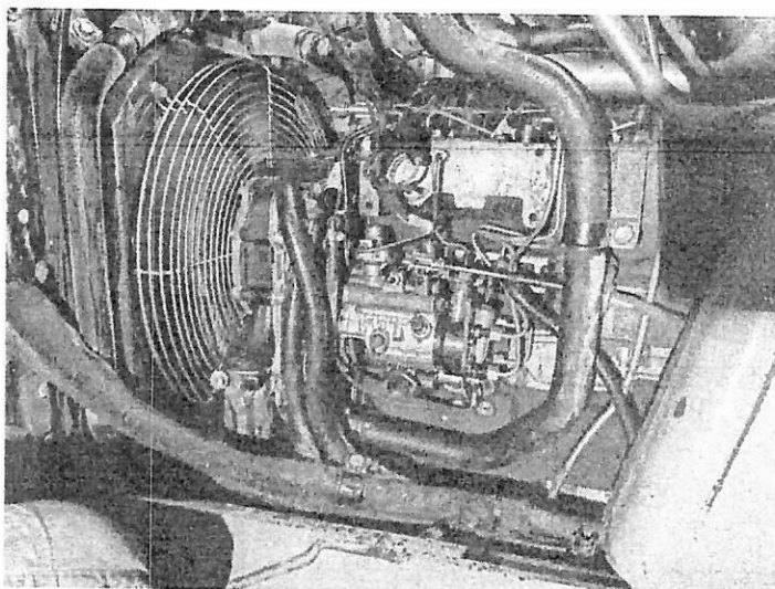
Bomba de inyección instalada y reparada Retrocargador 416E
