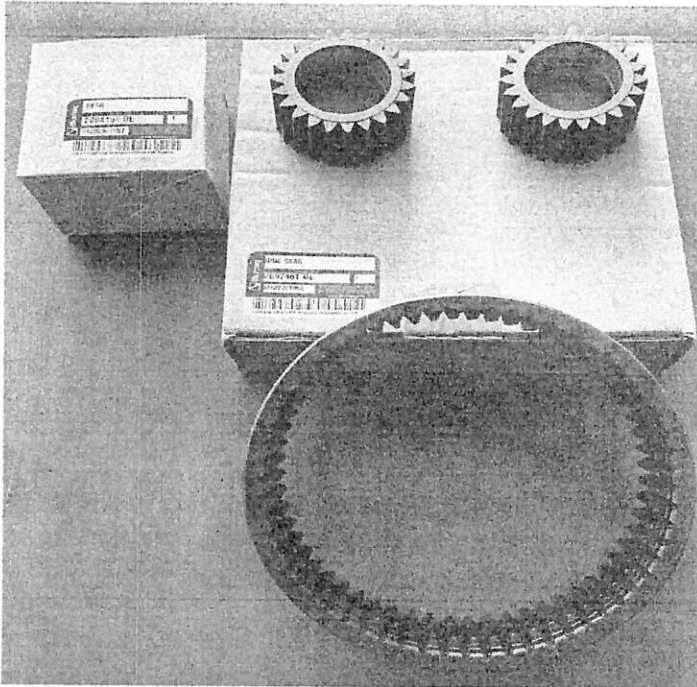
Corona y pillones de retrocargador 416E cambio por desgaste.
