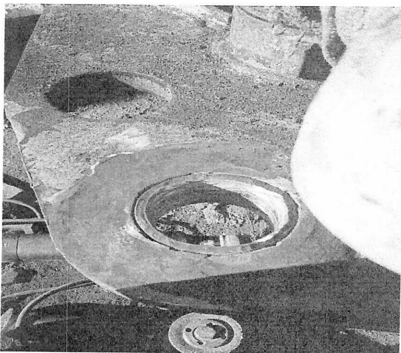
Relleno en soldadura a rotulas de retrocargador 416E
