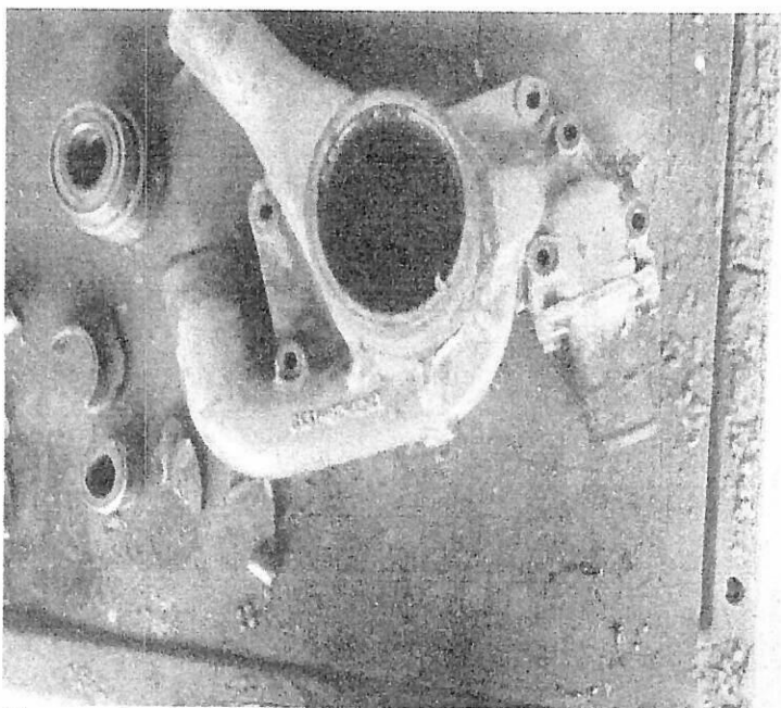
Reparacion bomba de agua de motoniveladora CAT 120K
