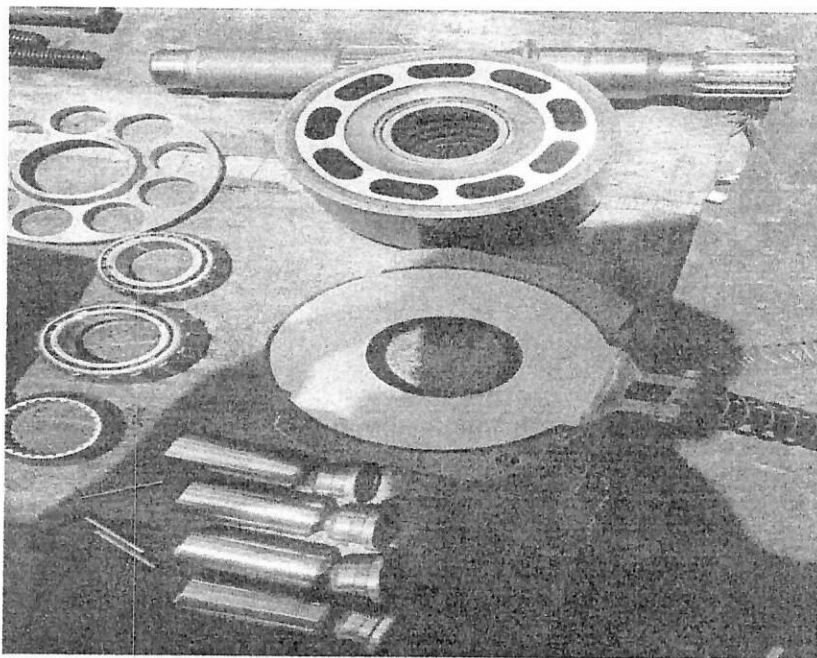
Mantenimiento bomba hidráulica retrocargador 416E
