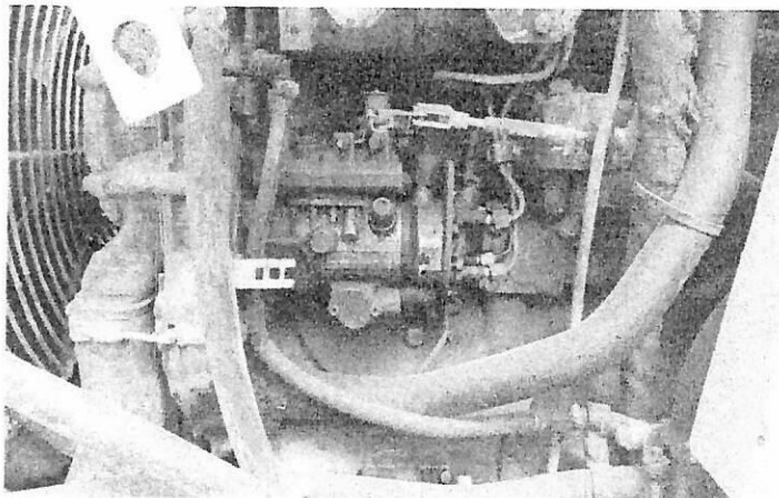
Bomba de inyeccion para reparar retrocargador 416E
