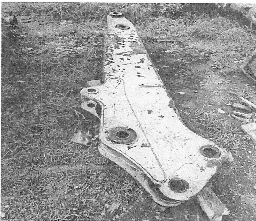
Desmante de pluma de retrocargador 416E
