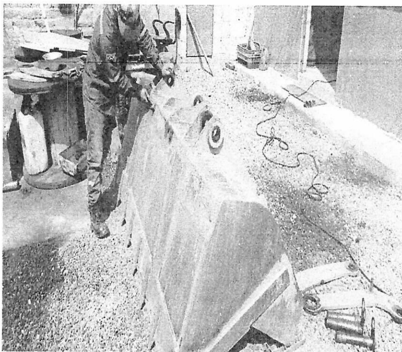
Reparaciones en soldadura a valde de retrocargador 416E
