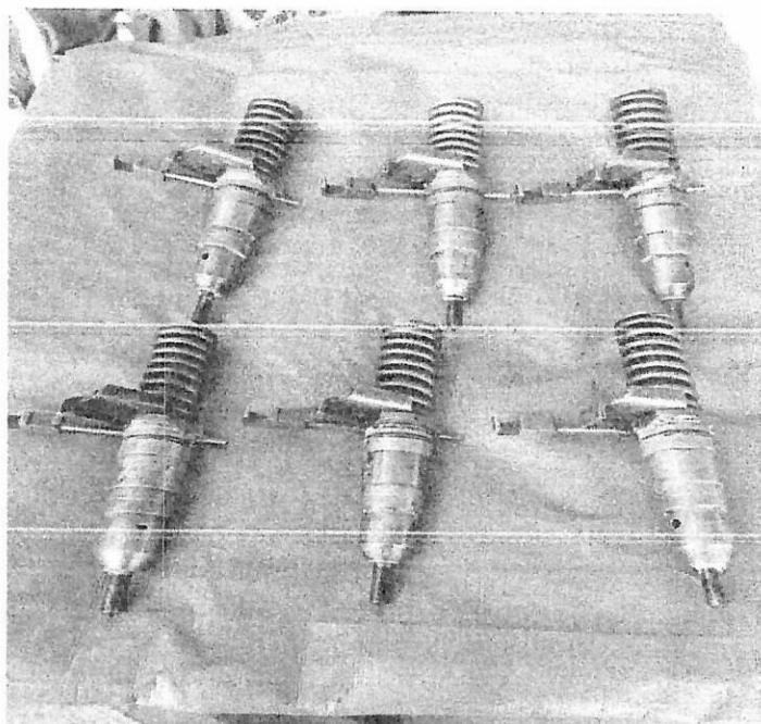
Desmonte de inyectores para mantenimiento de motoniveladora 120K.
