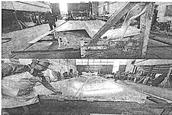
Foto No. 23 a 24 – Bote No. 24 quilla y láminas de fondo
