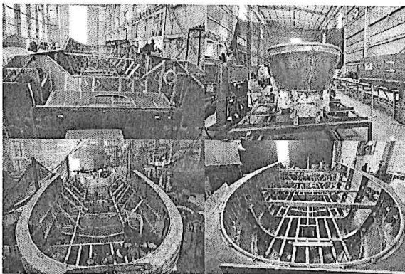
Foto No. 15 a 18 – Bote No. 19, 20, 21 y 22 forro del casco, refuerzos, tuberías y verduguillo
