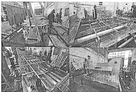
Foto No. 41 a 44 – Bote No. 24 refuerzos cuadernas vagras y tuberías
