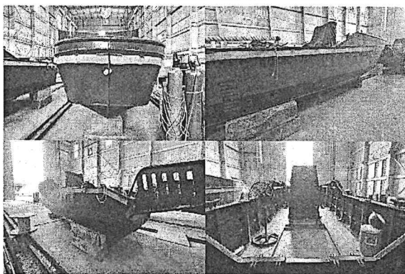
Foto No. 25 a 28 – Bote No. 13, 14, 15, 16 y 17 Espejo, refuerzos y tuberías.
