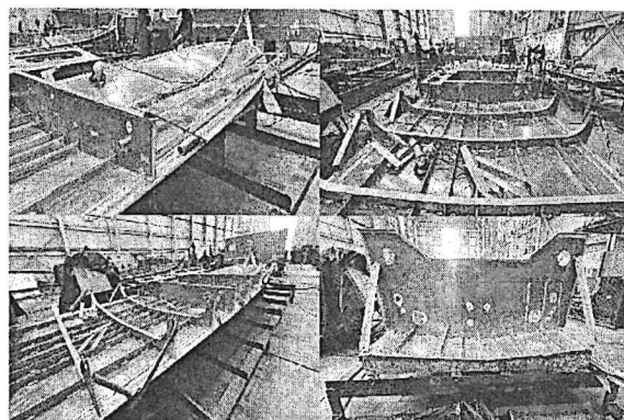
Foto No. 73 a 76 – Bote No. 26 refuerzos cuadernas y vagras
