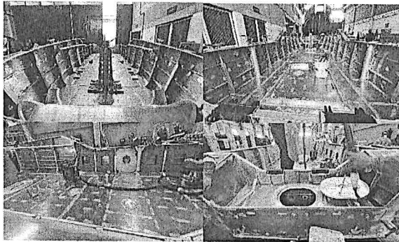
Foto No. 11 a 14 – Bote No. 17 y 18 cubierta, outfitting y soportes del balístico
