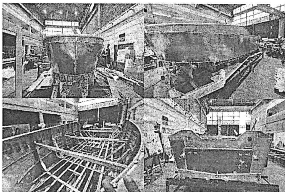
Foto No. 97 a 100 – Bote No. 24 refuerzos, forro del casco, tuberías, verduguillo y espejo
