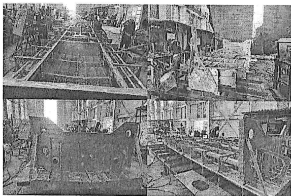
Foto No. 135 a 138 – Bote No. 26 refuerzos y tuberías
