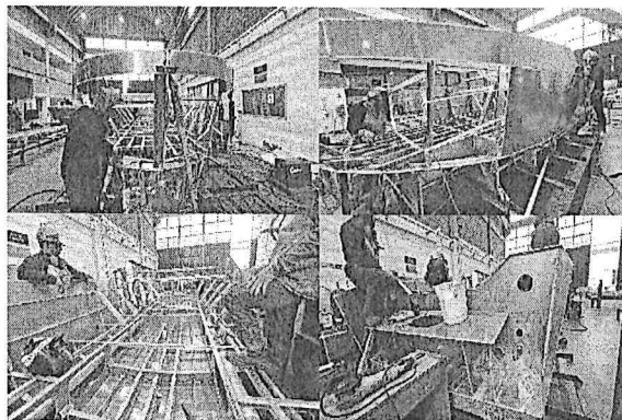
Foto No. 65 a 68 – Bote No. 24 refuerzos cuadernas, forro del casco y tuberías
