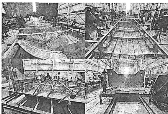
Foto No. 69 a 72 – Bote No. 25 cuadernas refuerzos y mamparos
