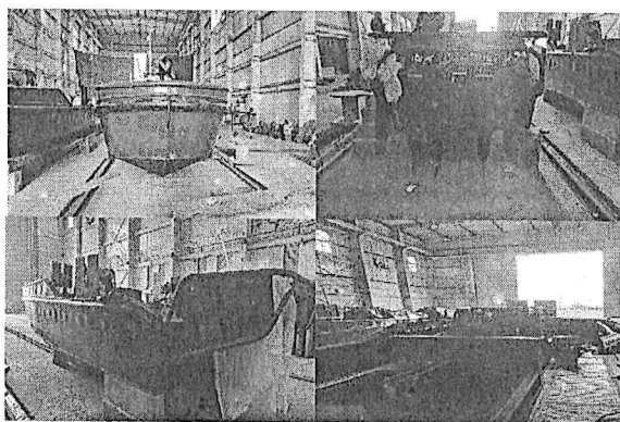
Foto No. 113 a 116 – Bote No. 17 y 18 equipos auxiliares y motores
