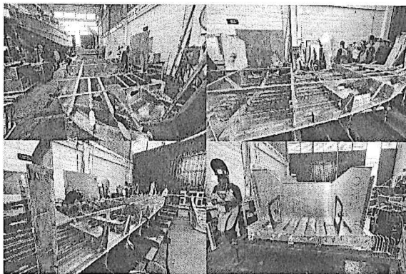
Foto No. 19 a 22 – Bote No. 23 refuerzos cuadernas y vagras
