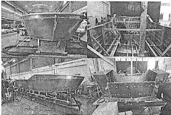
Foto No. 57 a 60 – Bote No. 19, 20, 21 y 22 volteo, END y cubierta principal
