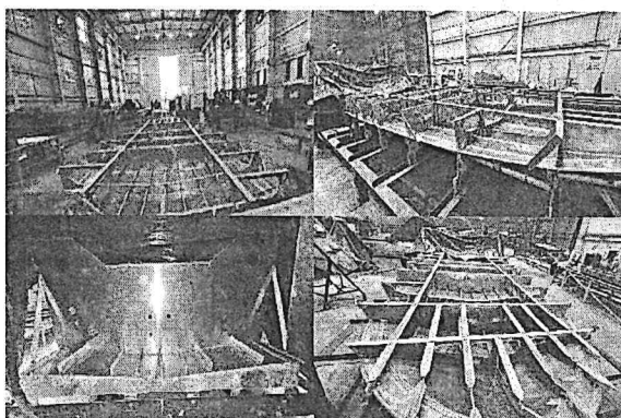
Foto No. 101 a 104 – Bote No. 25 refuerzos y cuadernas
