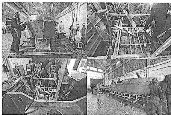
Foto No. 37 a 40 – Bote No. 23 refuerzos forro del casco
