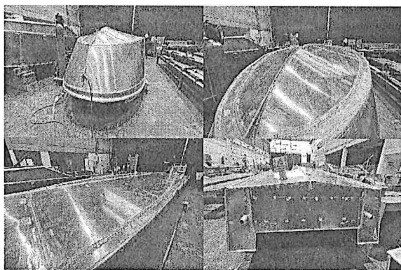
Foto No. 93 a 96 – Bote No. 23 volteo
