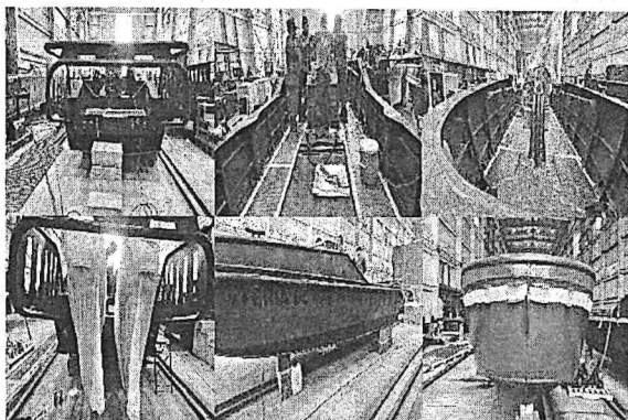
Foto No. 51 a 56 – Bote No. 13, 14, 15, 16, 17 y 18 equipos, defensas, balístico afustes y motores
