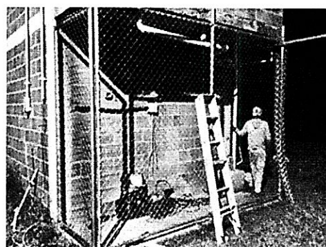
Foto No. 18 CERRAMIENTO MALLA ESLABONADA ZONA TANQUES CLORO Y SULFATO
