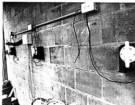
Foto No. 16 SISTEMA BOMBAS DOSIFICADORAS CLORO Y SULFATO
